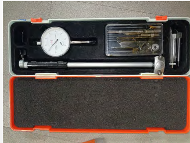
内径ダイヤルゲージ
